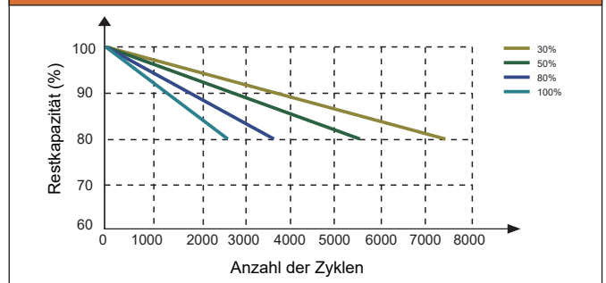
UNTERSCHIEDLICHE DOD-ENTLADUNGSZYKLUS-LEBENS-KURVE
