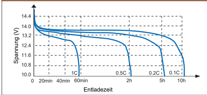
ENTLADEKURVE MIT UNTERSCHIEDLICHER RATE (25°C)
