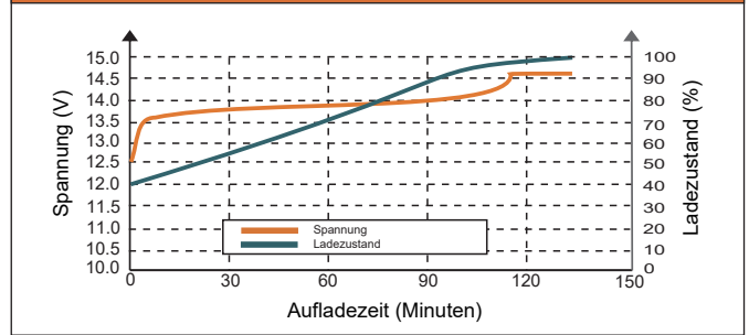
LADEZUSTANDSKURVE (0.5C, 25°C)
