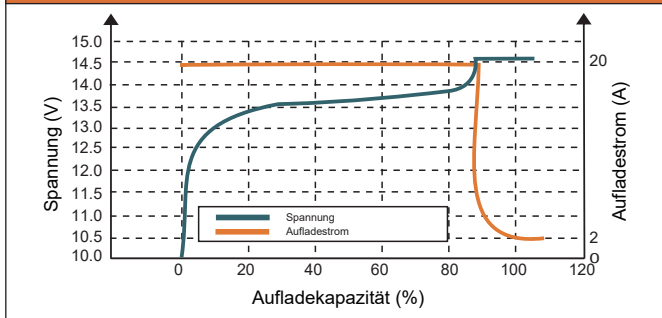
LADECHARAKTERISTIK (0.5C, 25°C)
