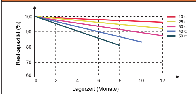
UNTERSCHIEDLICHE TEMPERATUR-SELBSTENTLADEKURVE
