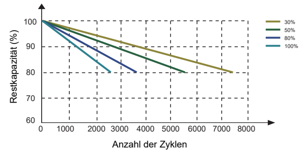
UNTERSCHIEDLICHE DOD-ENTLADUNGSZYKLUS-LEBENSKURVE
