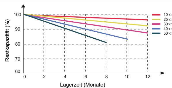
UNTERSCHIEDLICHE TEMPERATUR-SELBSTENTLADEKURVE
