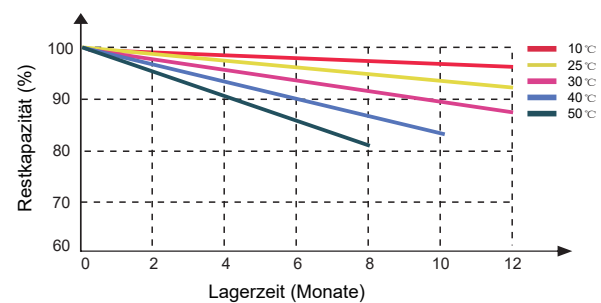
UNTERSCHIEDLICHE TEMPERATUR-SELBSTENTLADEKURVE
