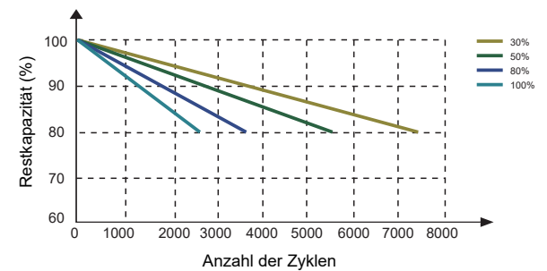
UNTERSCHIEDLICHE DOD-ENTLADUNGSZYKLUS-LEBENS-KURVE
