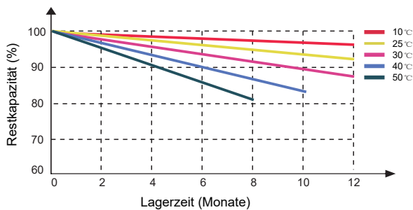
UNTERSCHIEDLICHE TEMPERATUR-SELBSTENTLADEKURVE
