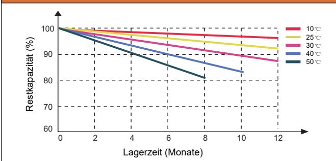
UNTERSCHIEDLICHE TEMPERATUR-SELBSTENTLADEKURVE
