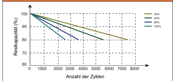
UNTERSCHIEDLICHE DOD-ENTLADUNGSZYKLUS-LEBENS-KURVE
