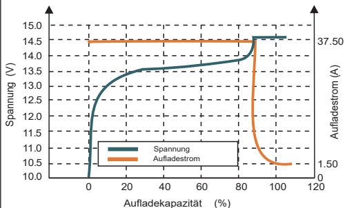
Ladecharakteristik (0,5C, 25°C)
