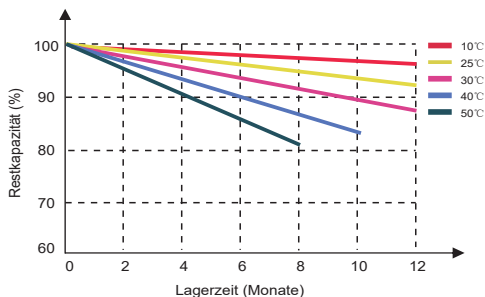
Unterschiedliche Temperatur-Selbstentladekurve
