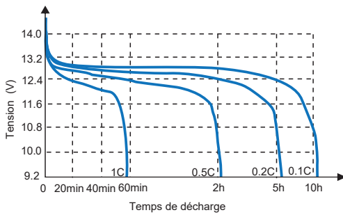
Courbe de décharge à différents taux (25 °C)
