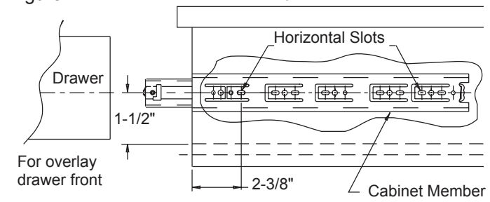
Figure 2 32 mm System—Cabinet
