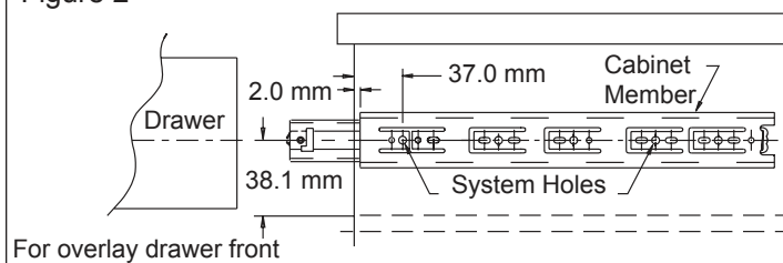
Figure 2 32 mm System—Cabinet
