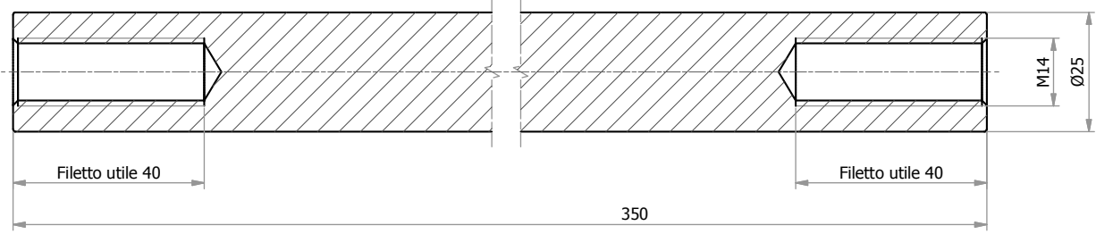
Sez. A-A Scala 1:1
