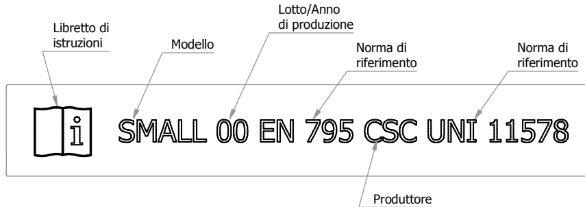
Dettaglio marcatura scala 1:1
