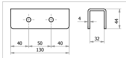
Dettaglio "C" Scala 1:3
