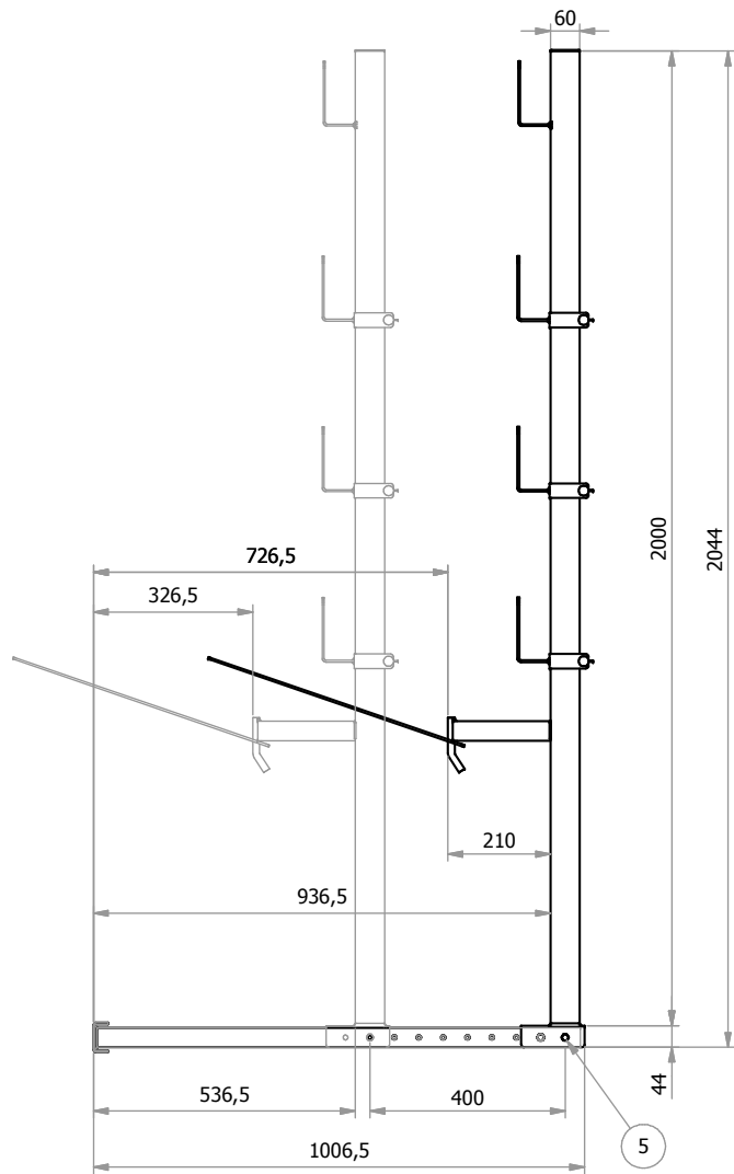
Dettaglio A Scala 1 : 6
