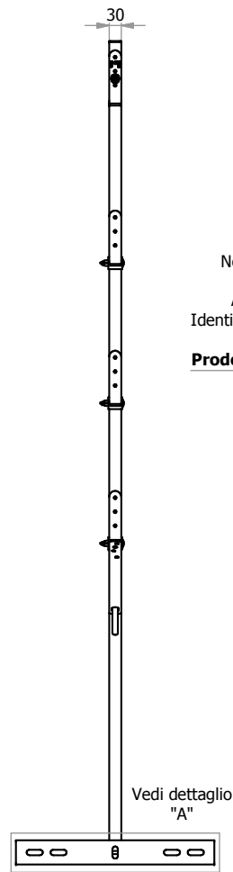
Dettaglio "C" Scala 1:3
