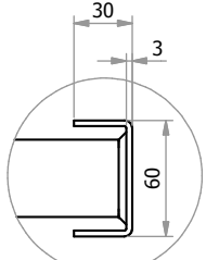
Dettaglio B Scala 1 : 3
