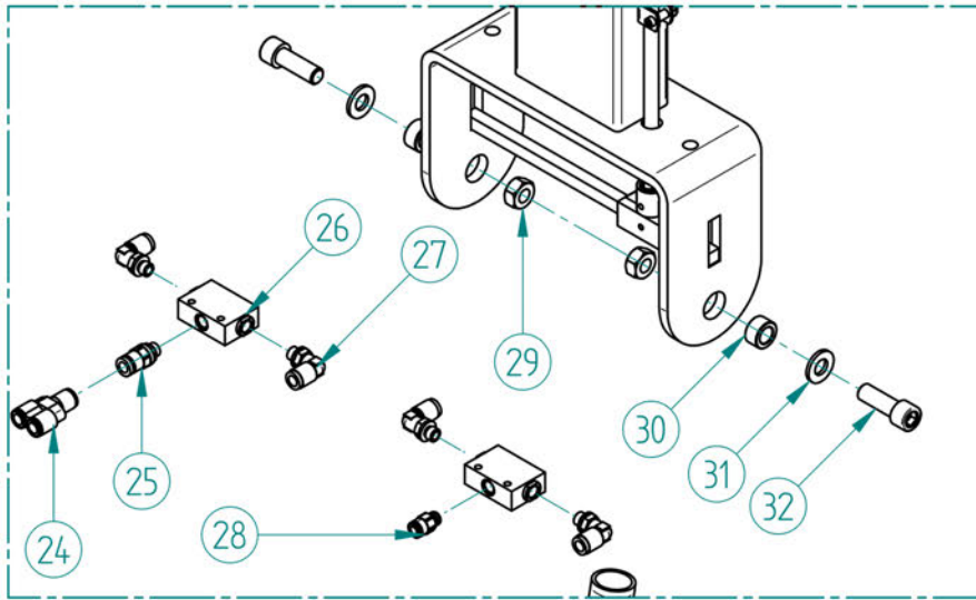
DETTAGLIO A
