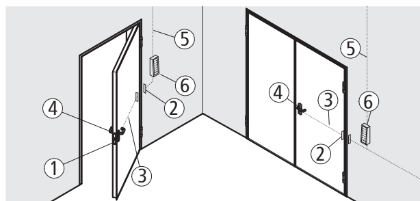
Schema componenti
