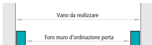
Sezione orizzontale
