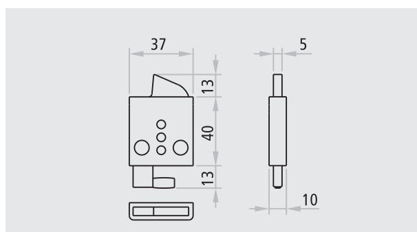
Dispositivo superiore per anta passiva UNIVER e REVER
