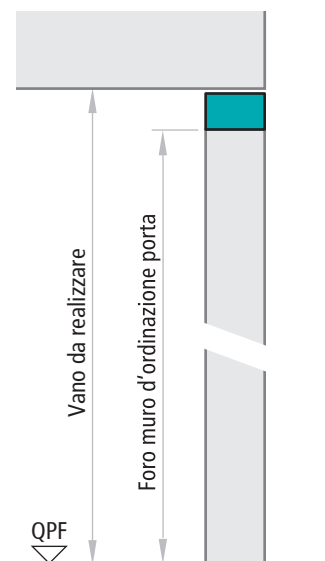
Sezione verticale
