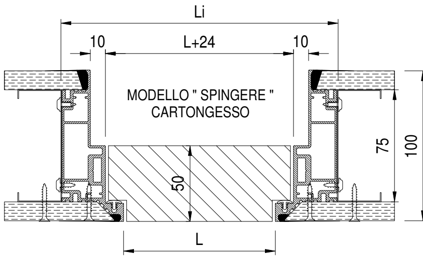
SEZIONE ORIZZONTALE
