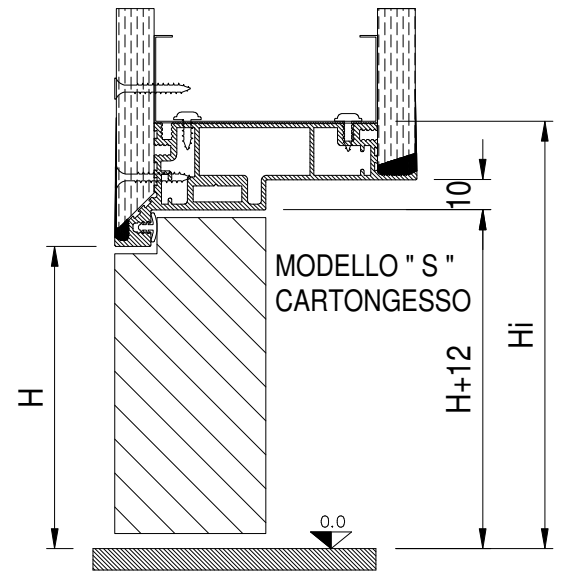
SEZIONE VERTICALE
