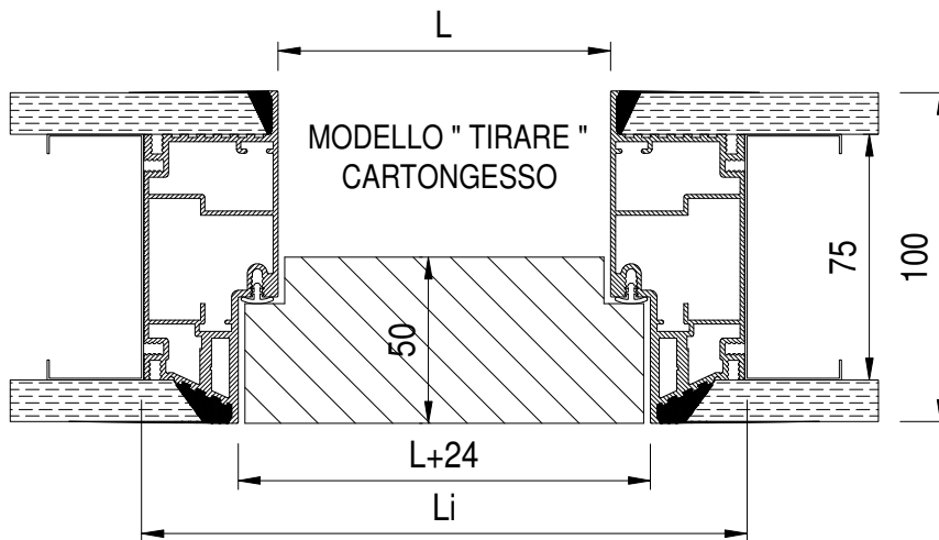
SEZIONE ORIZZONTALE
