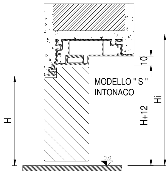
SEZIONE VERTICALE
