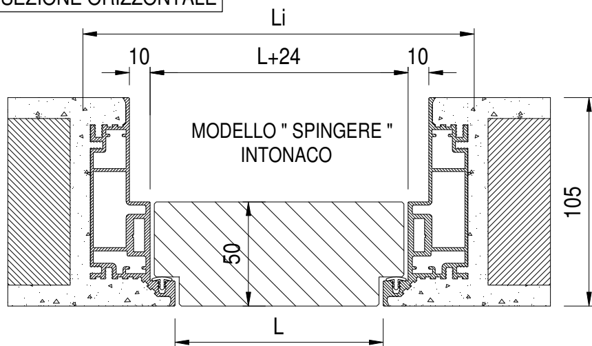
SEZIONE ORIZZONTALE
