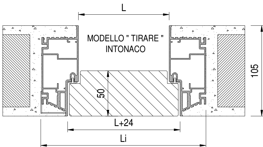
SEZIONE ORIZZONTALE
