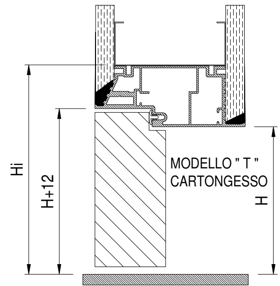
SEZIONE VERTICALE
