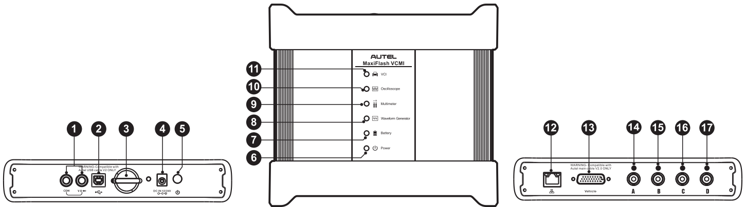
MaxiFlash VCM1
