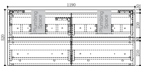
MIA 120DW Front Section
