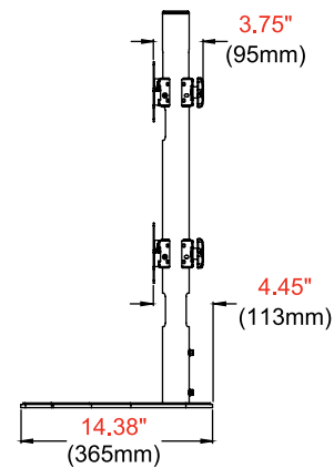
SEITENANSICHT
