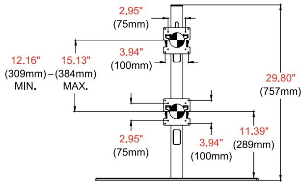
VORDERANSICHT
