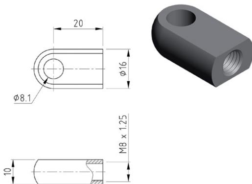
PART NO: AL03
