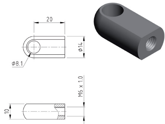
PART NO: AL04
