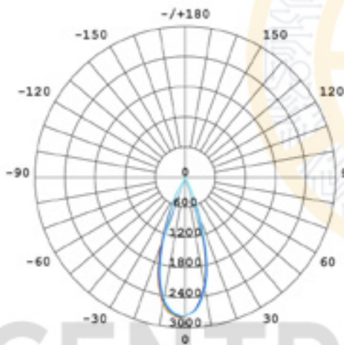
Curva fotométrica
