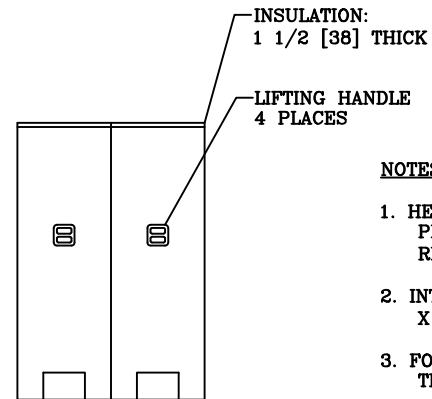
VIEW A-A
