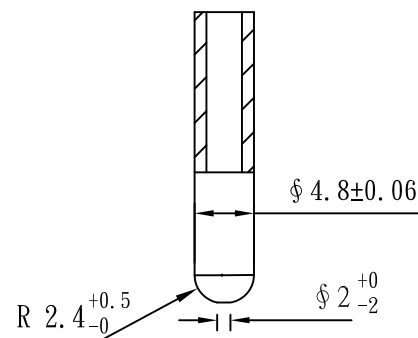
PIN的尺寸
