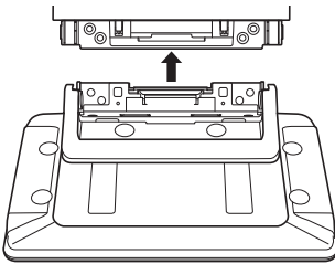
Винты (M5×8) (в комплекте)
