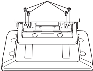
Винты (M5×8) (в комплекте)
