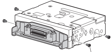
Sechskantschrauben (x4)
