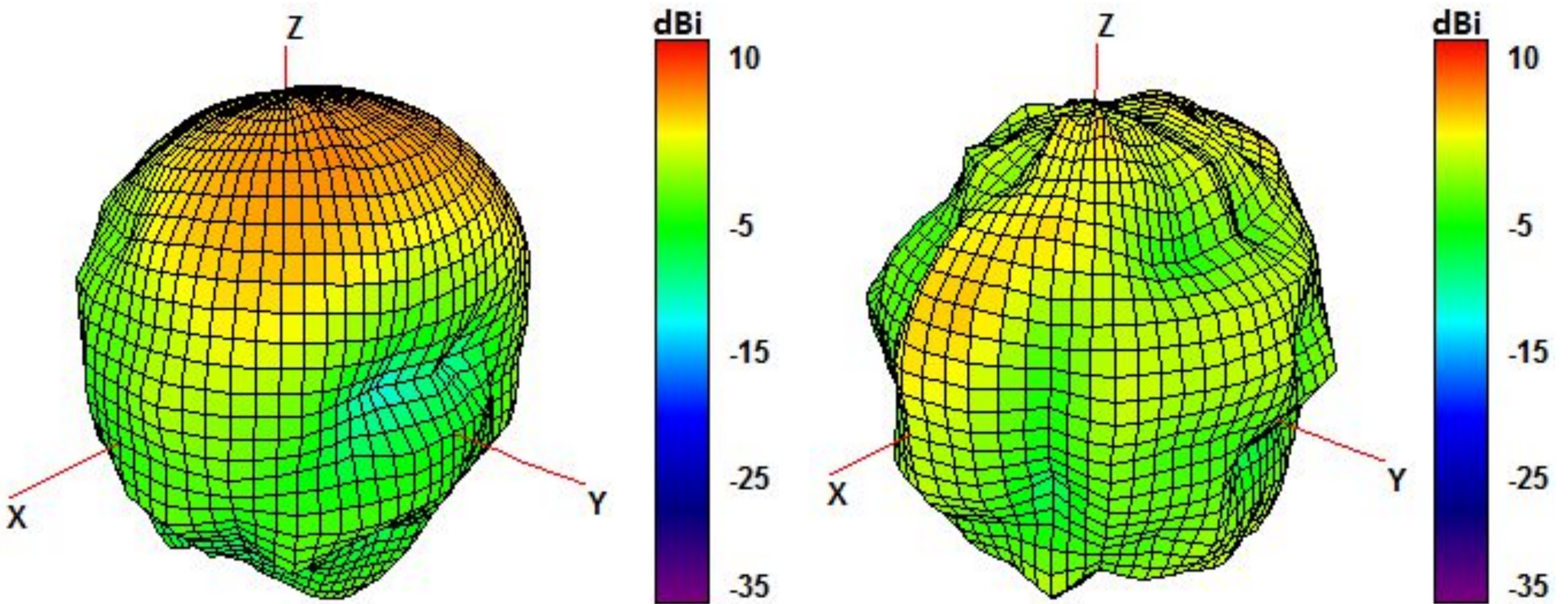
Cable 3: 2.4/5.0 GHz ISM
