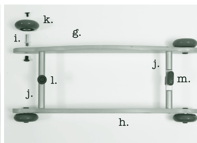
Mini-Flip-Inline-Unterteil
