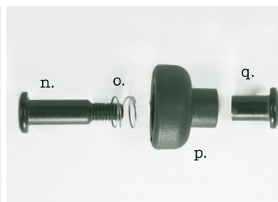
Gleitknopfbaugruppe
