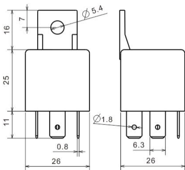
外形尺寸 Outline Dimensions
