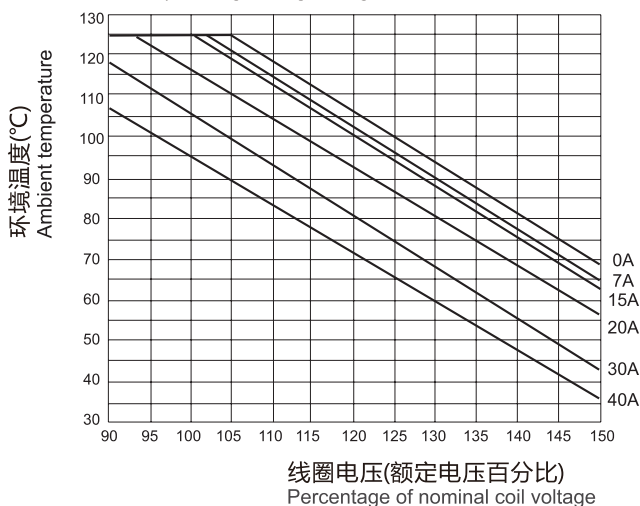
2. 允许最大负载范围(23°C) Load Limit Curve
