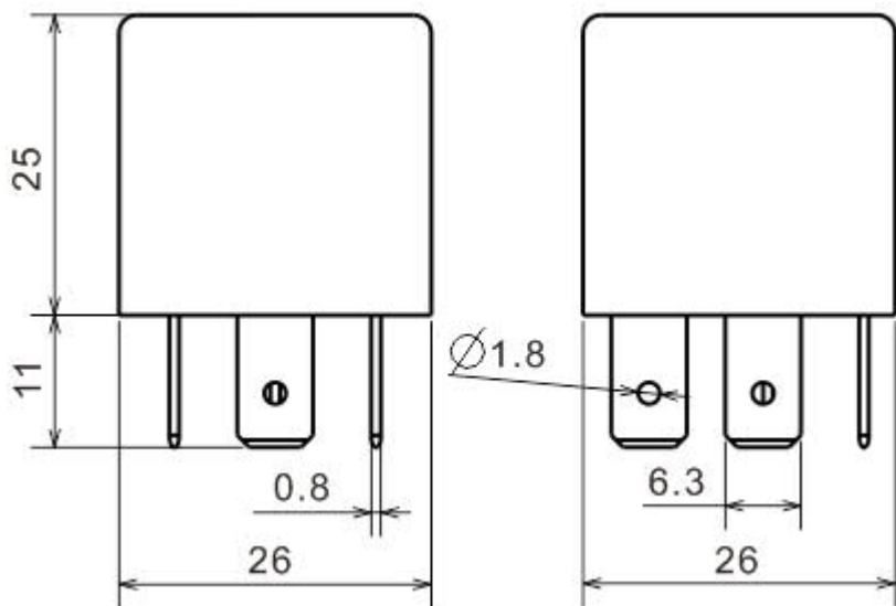
外形尺寸 Outline Dimensions
