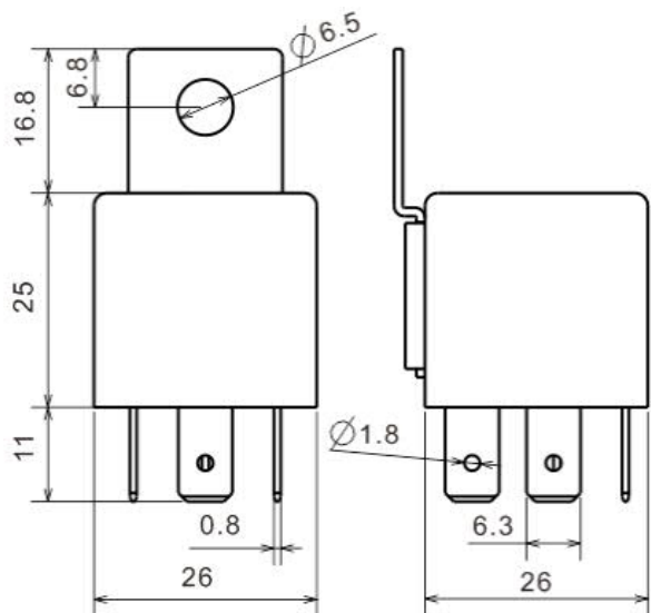
外形尺寸 Outline Dimensions
