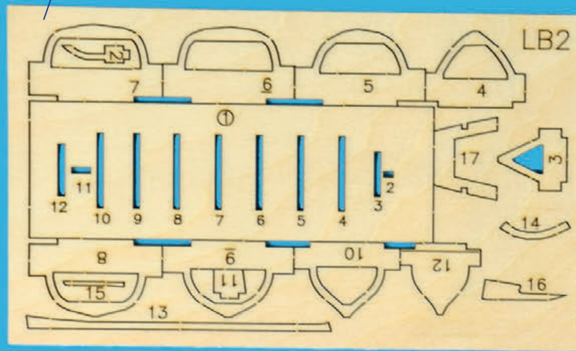
LB2 1,5 mm plywood
