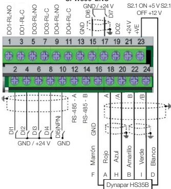
(b) Señales del conector de control para el módulo CFW500-ENC2
