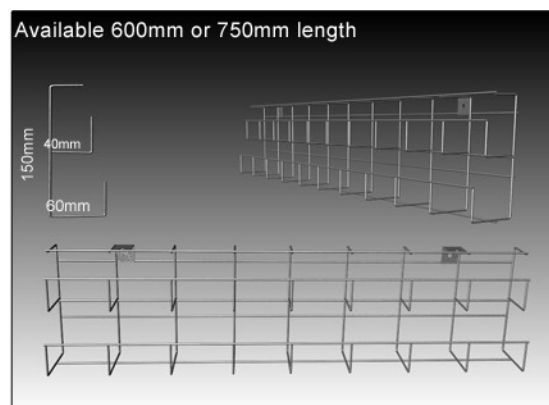
Cable Tray - ODCT6 600mm - ODCT7 750mm
