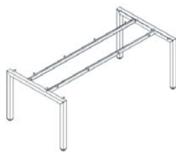
Plaza Table Frame IMPLFM
