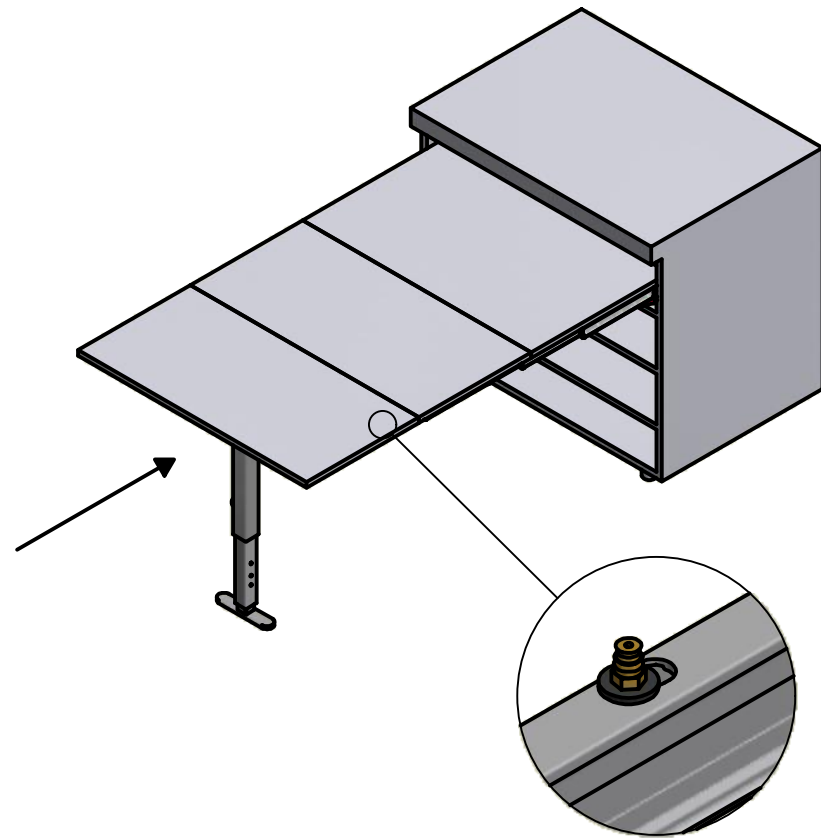
APERTO, SPINGERE LE GAMBE VERSO L'INTERNO OPENED, PUSH THE LEG TOWARDS THE CABINET
