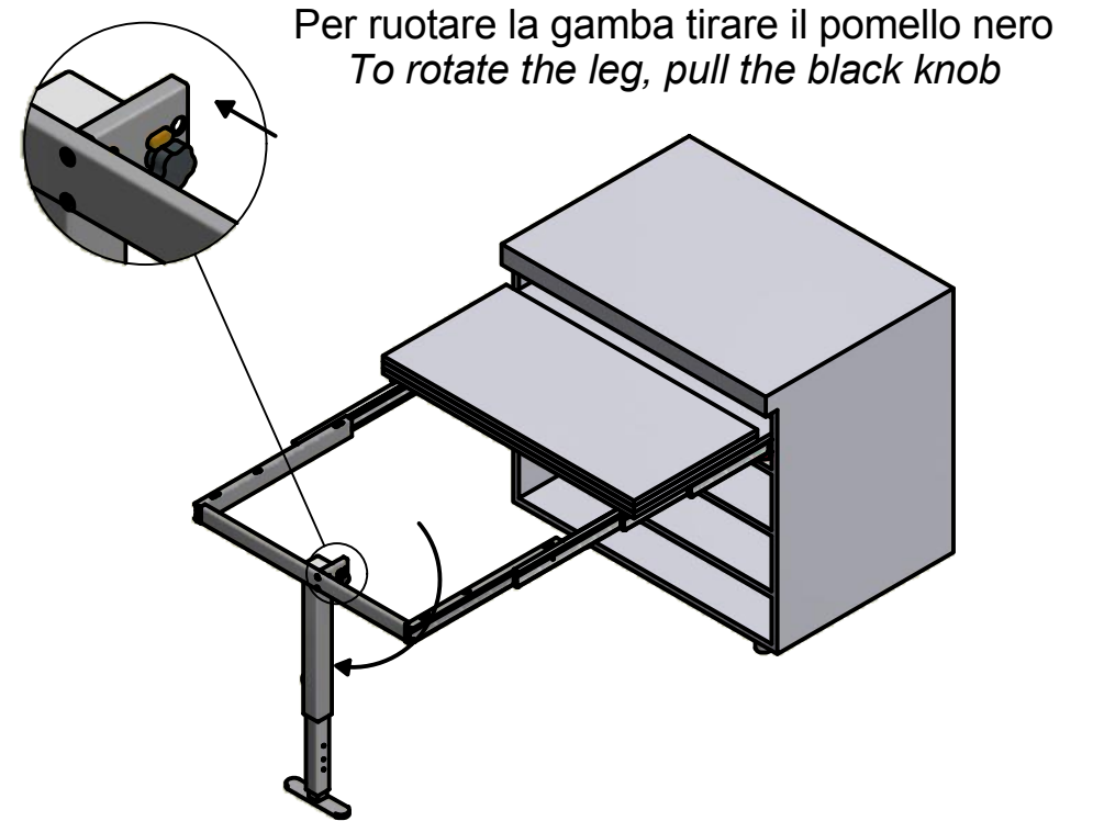
SBLOCCO E ROTAZIONE DELLA GAMBA LEG RELEASE AND ROTATION Per ruotare la gamba tirare il pomello nero To rotate the leg, pull the black knob
