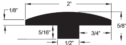
78" T-Mold
