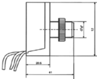
Exterior dimension(mm)
