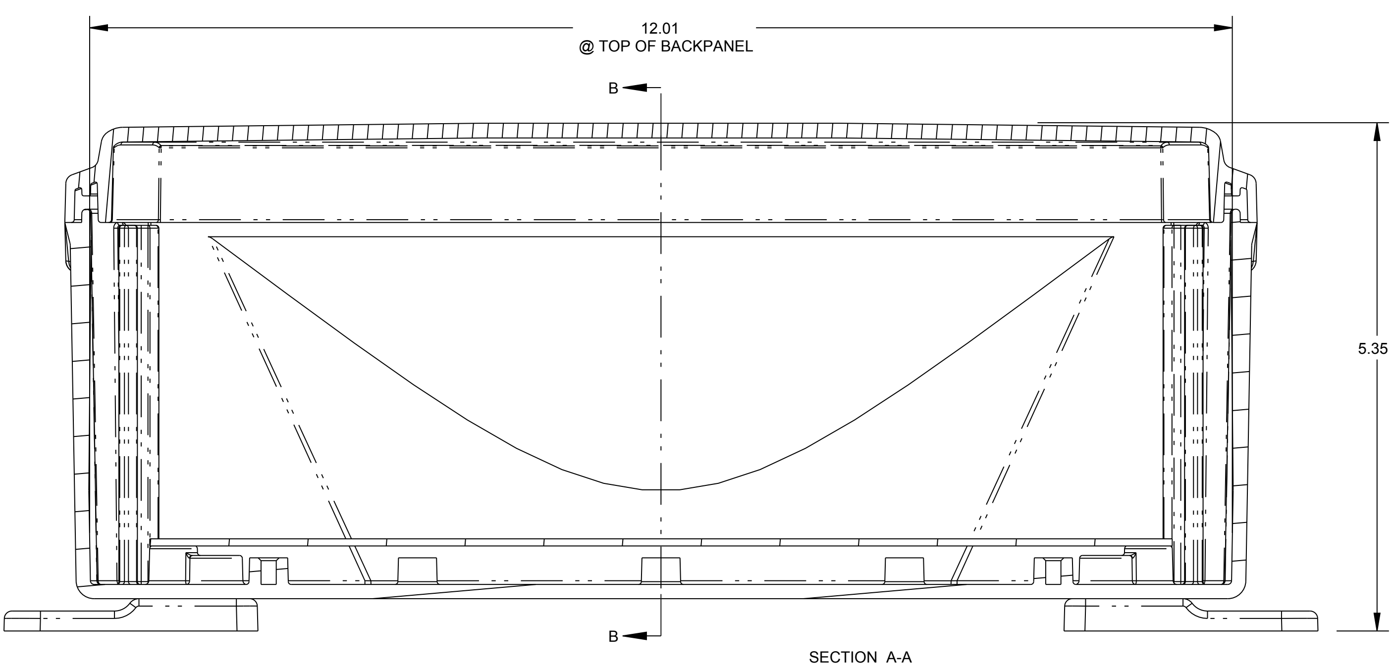
SECTION A-A
