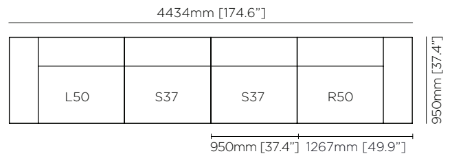
Modular 4 Sofa BLD.MS.CON.S4
