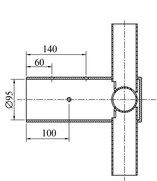
B-B
