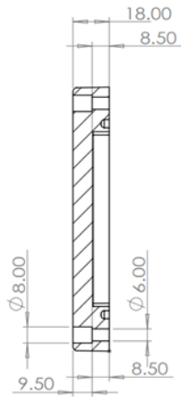
A-A
