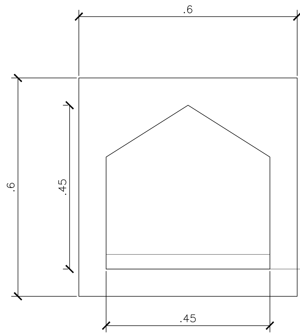
VISTA FRENTE
