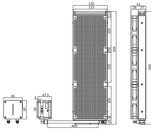
ELC-LMT360-W-ARGB
