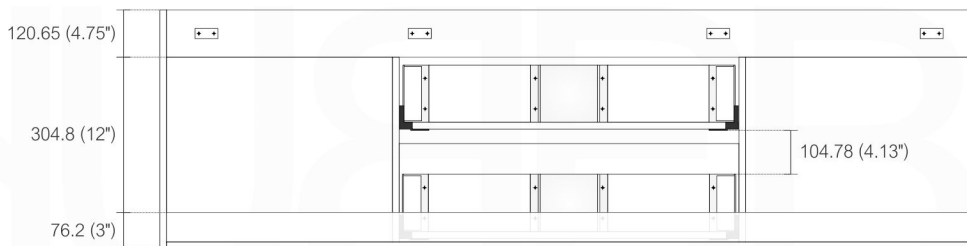
. TOP ELEVATION
