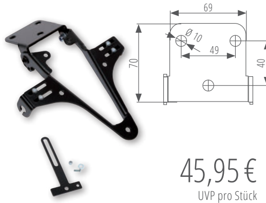
HIGHSIDER™ Kennzeichenhalter Universalhalter Typ 3 Art.-Nr.: 280-203
