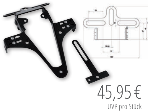
HIGHSIDER™ Kennzeichenhalter Universalhalter Typ 6 Art.-Nr.: 280-206
