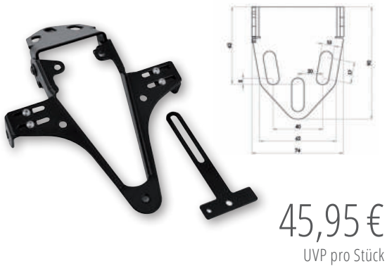
HIGHSIDER™ Kennzeichenhalter Universalhalter Typ 5 Art.-Nr.: 280-205
