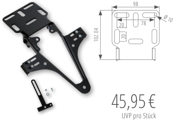
HIGHSIDER™ Kennzeichenhalter Universalhalter Typ 2 Art.-Nr.: 280-202
