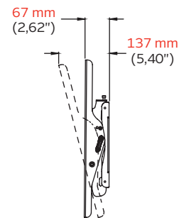
VUE LATÉRALE INCLINAISON DE +15°/-5°
