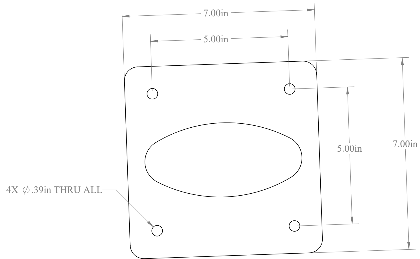
VIEW A-A
