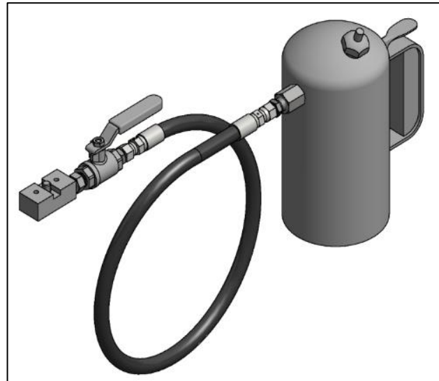
Figure 18: 1 QT Mini Flush Tank (200216)
