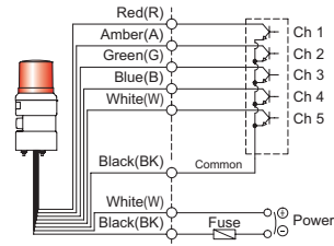
STND100DL-DC/AC
