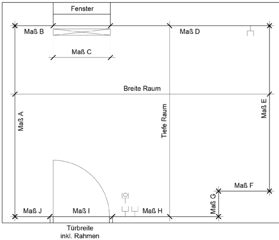
AUFMAß GRUNDRISS RAUM
