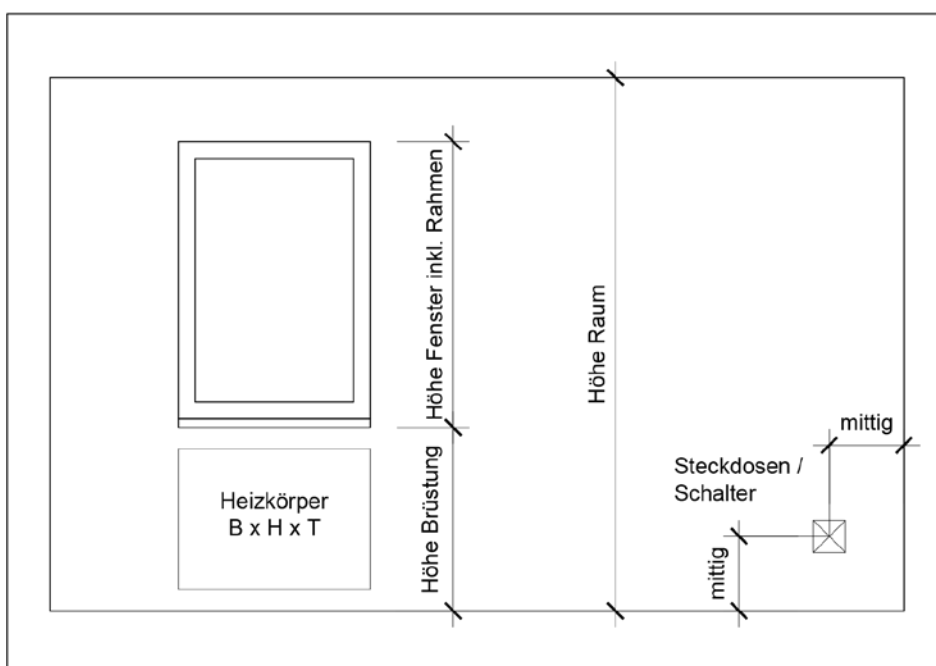
AUFMAß ANSICHT WAND
