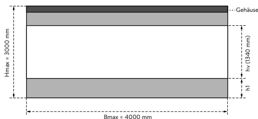
Typ 1 Durchgehendes Fenster über die ganze Breite
