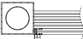
zijprofiel met schuifgrendel CGHS
