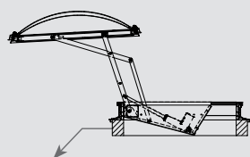
avec costière en PVC 16/00 ou PVC 20/00 hauteur totale min 300 mm
