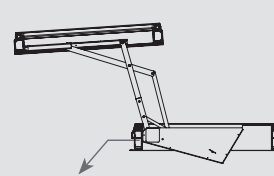
avec costière en PVC 20/00
