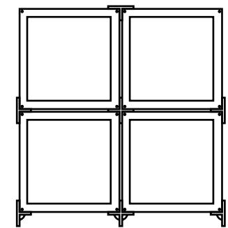
BUNKE (4x opslag + 4x verbindingskruis + 10x verbinding zijkant)
